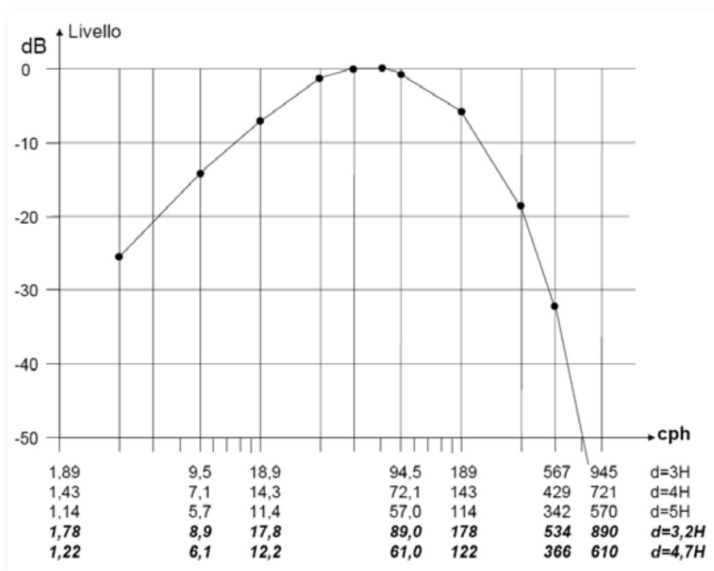
Fig. A2 – Funzione di trasferimento del sistema visivo umano a distanze di visione di 3H; 4H; 5H; 3,2H e 4,7H, dove H indica l'altezza dello schermo. Gli ultimi due valori di distanza di visione corrispondono alle distanze limite che consentono una percezione di tutta la risoluzione disponibile con immagini HDTV 1080i/p e 720p. Le frequenze sono indicate in cicli per altezza di schermo (cph); moltiplicando il valore per 16/9 si ottengono le frequenze orizzontali misurate in cpw.
