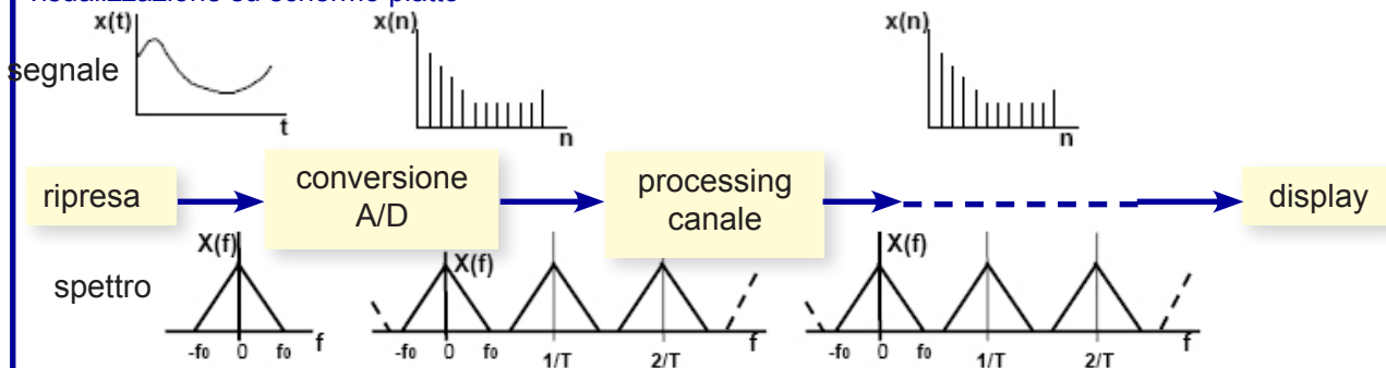
Fig. 1 – Schematizzazione della catena “dalla generazione alla visualizzazione” nel caso di display a raggi catodici (CRT) ed a schermo piatto (LCD, PDP, ecc.). Gli schermi a raggi catodici (CRT) ricevono al loro ingresso un segnale analogico e, trascurando l'effetto della maschera, si può ritenere che questi visualizzino l'immagine in modo continuo nella direzione orizzontale dello schermo. Gli schermi piatti ricevono invece un segnale campionato, costituito da 1920x1080 o 1280x720 campioni immagine rispettivamente orizzontali e verticali, e devono convertire tali formati nel numero di pixel orizzontali e verticali dello schermo mediante un'operazione detta di interpolazione. Inoltre, benché nelle odierne telecamere a CCD o CMOS la digitizzazione venga effettuata dal CCD/CMOS stesso, in figura è riportato il blocco A/D al fine di evidenziare l'effetto di tale operazione sullo spettro dell'immagine.
