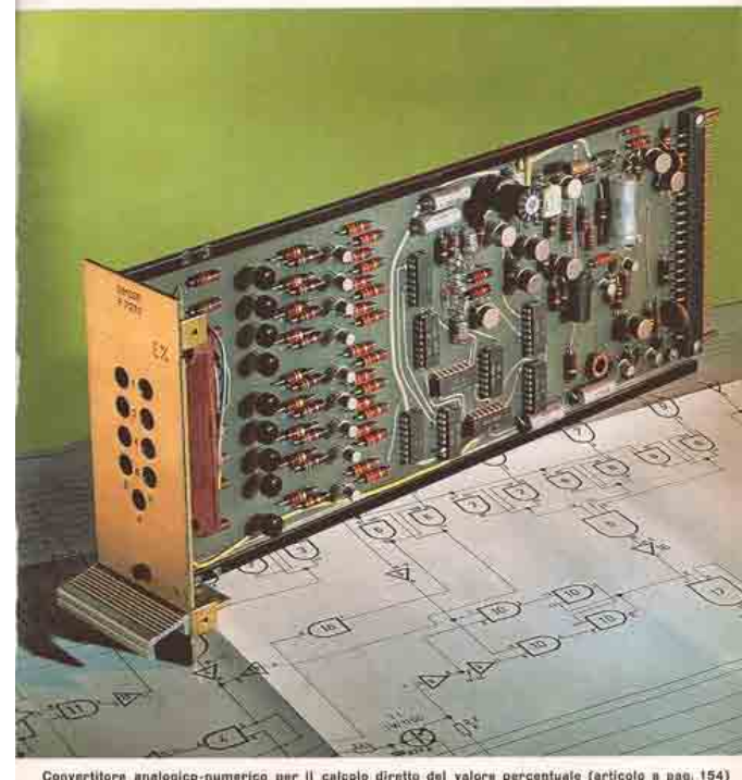
Convertitore analogico-numeric per il calcolo diretto del valore percentuale (articolo a pag. 154)
