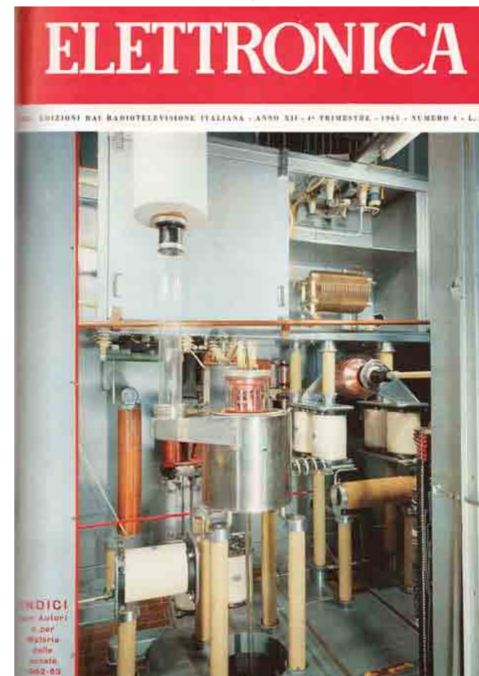
4. Uno dei tubi con raffreddamento a vapore dello stadio finale del trasmettitore ad onda media da 100 chilowatt di Firenze 1, recentemente rammodernato.
