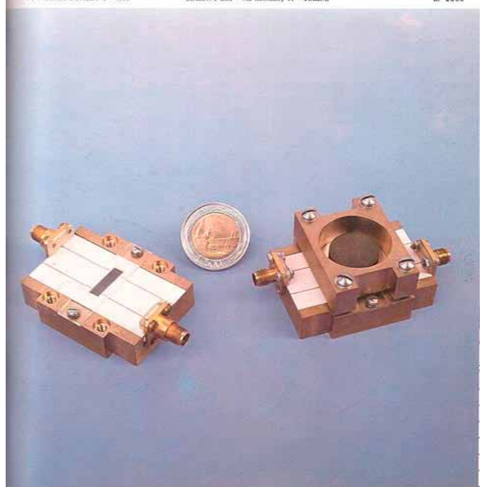
Prototipi di linea di ritardo dispersiva lineare ad onde magnetostatiche (Selenia, IESS-CNR - v. p. 206)
