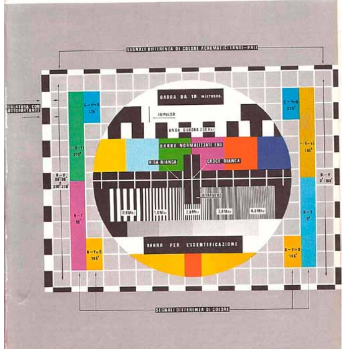
Immagine del monoscopio elettronico a colori Philips con scritte illustrative (v. articolo a pag. 211).
