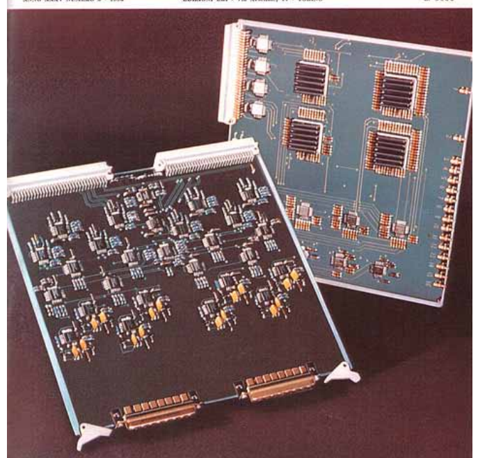
Circuiti per la commutazione di segnali a 140 Mbit/s per servizi a larga banda (v. p. 105).
