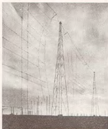
CENTRO TRASMETTENTE A ONDE CORTE ROMA-PRATO SMERALDO: Veduta di una parte delle antenne.
