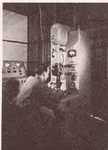
Oscillografo a catodo freddo a due raggi per rilevamento di transistori rapidi, presso la Sezione Alta Tensione dell'Istituto Elettrotecnico Nazionale G. Ferraris di Torino.
